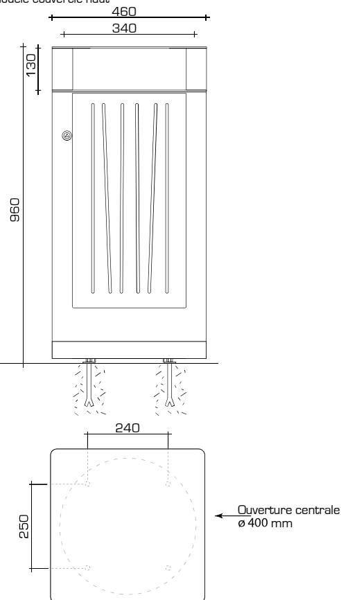
Mod le couvercle haut
