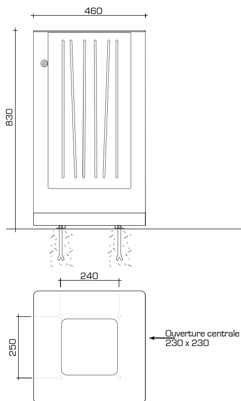
Mod le couvercle bas
